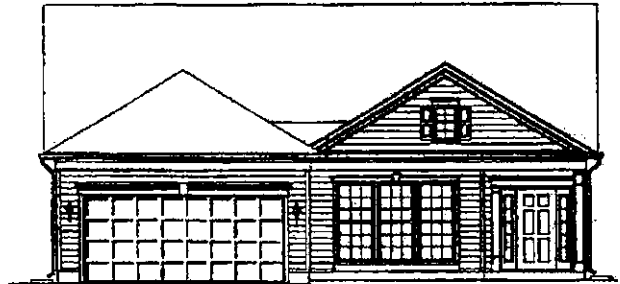
ELEVATION 3
